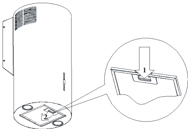
Рис.11 Снятие жиро-улавливающего алюминиевого фильтра
