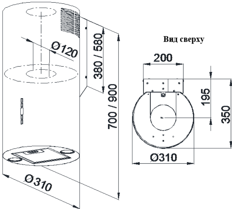
Рис. 2 Схема габаритов
