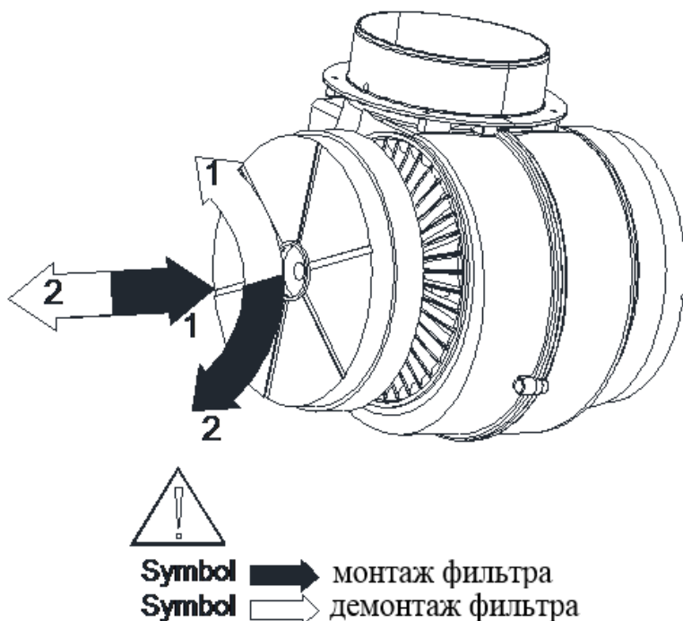
Рис.12 Установка и снятие угольного фильтра
